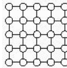
Рис. 1: Система соседства — прямоугольная решетка
